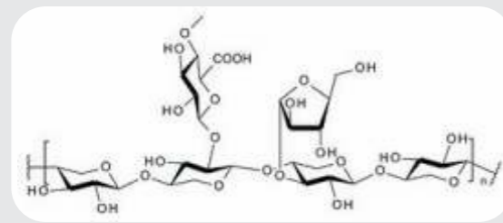
آرابینوزایلان
