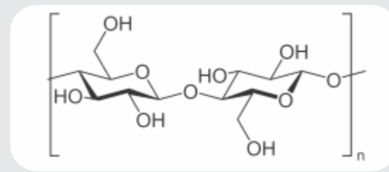
سلولز
