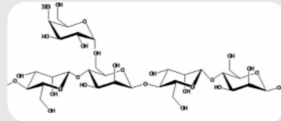
گالاکتومانان
