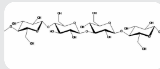
گلوکومانان
